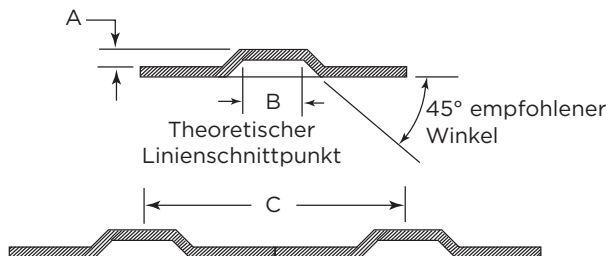
Kragenprägung
