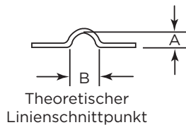
Schweissbuckel
